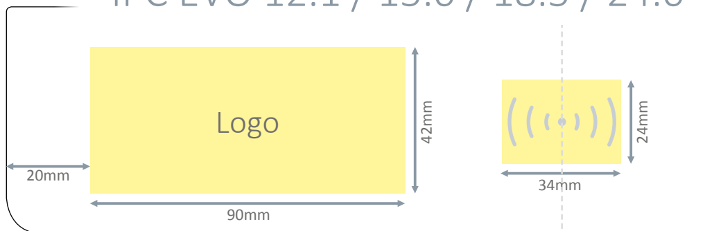
Beispiel Sensorglas des Datafox IPC EVO 12.0
