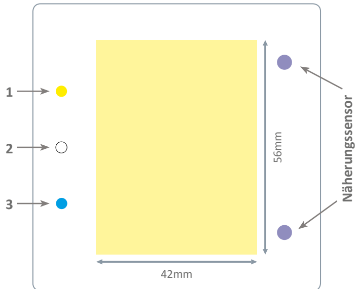
Das Frontglas des EVO Intera II kann mit der Leuchtfäche hochformatig gestaltet werden.
